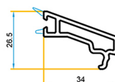
PR.OF.99.BL/514 Parcloses simple vitrage
