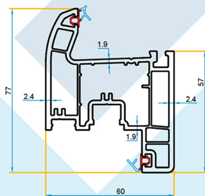
PR.OF.02.BL/104 Ouvrant fenêtre Blanc
