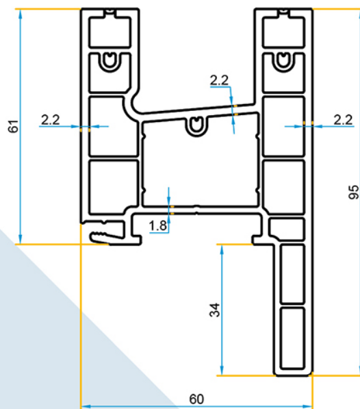
PR.OC.22.BL/225 Dormant avec aile de recouvrement Blanc
