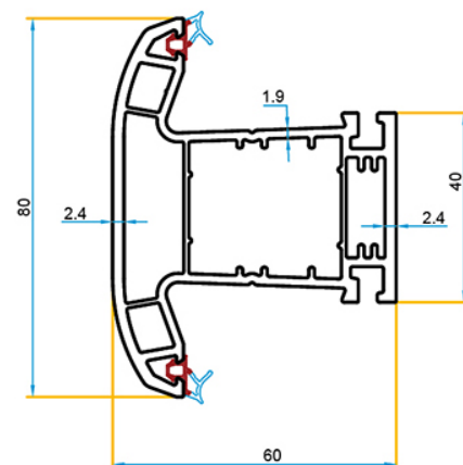
PR.OF.03.BL/107 Traverse/ Meneau
