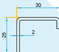
S-634TRE01 Renfort ouvrant Fenêtre
