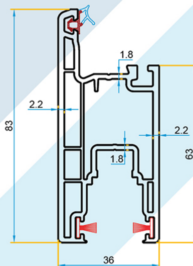
PR.OC.24.BL/107 Ouvrant porte fenêtre 36/83 Blanc
