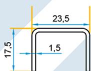
S-634TRE16B Renfort ouvrant Fenêtre
