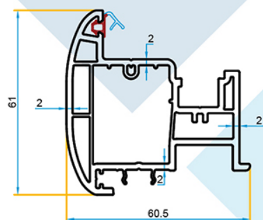
PR.OF.04.BL/108 Battée extérieure Blanc
