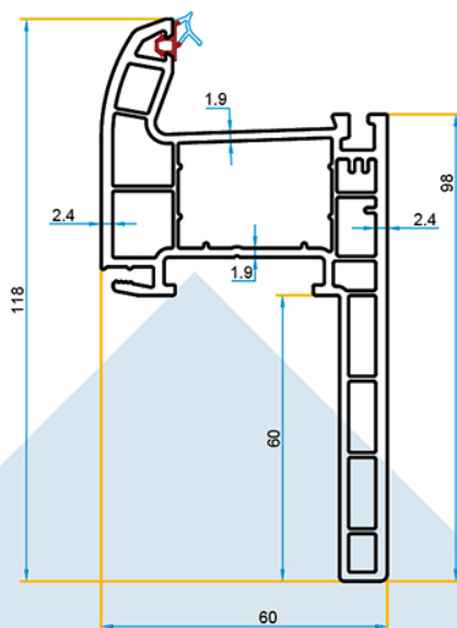
PR.OF.95.BL/103 Dormant avec recouvrement Blanc
