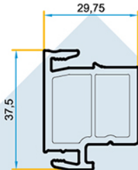
PR.FC.21.BL PROFILE ELARGISSEUR REHAUSSEUR
