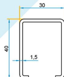
S-634TRE04 Renfort ouvrant Porte-fenêtre
