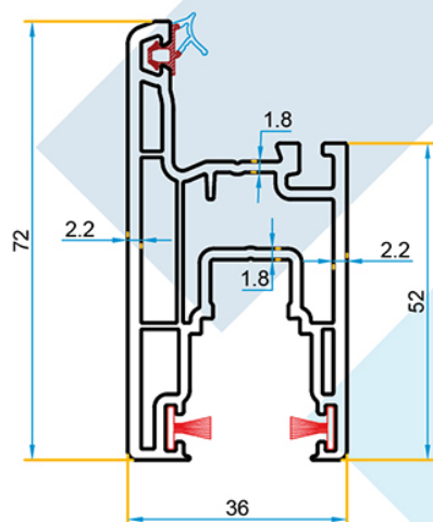
PR.OC.23.BL/106 Ouvrant fenêtre 36/72 Blanc
