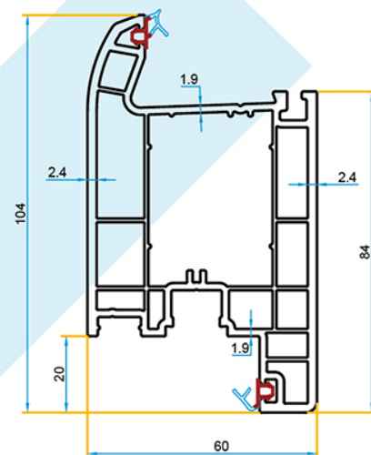
PR.OF.08.BL/105 Ouvrant porte Blanc
