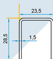
S-634TRE17B Renfort ouvrant Porte-fenêtre
