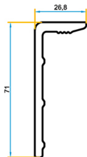
PR.FC.24.BL AILETTE D'HABILLAGE
